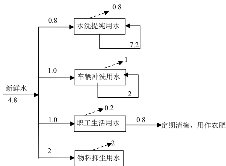
图 1 全厂给排水平衡图 (m³/d)
