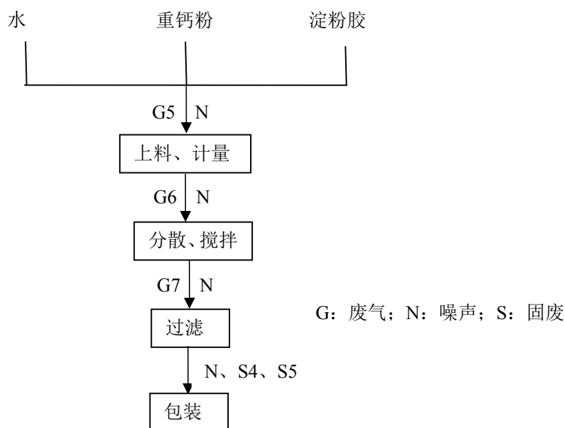
图 4 防火材料（液体）工艺流程及产排污环节示意图
