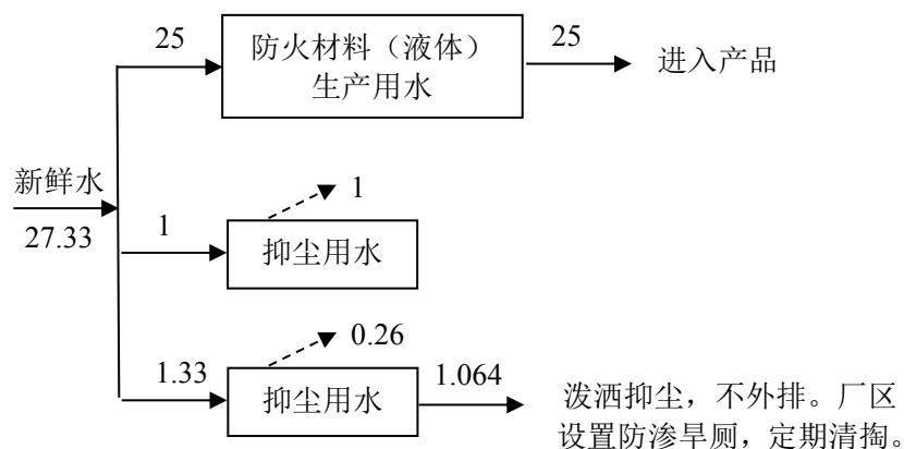
图 1 项目给排水平衡图 单位：m 3 /d
