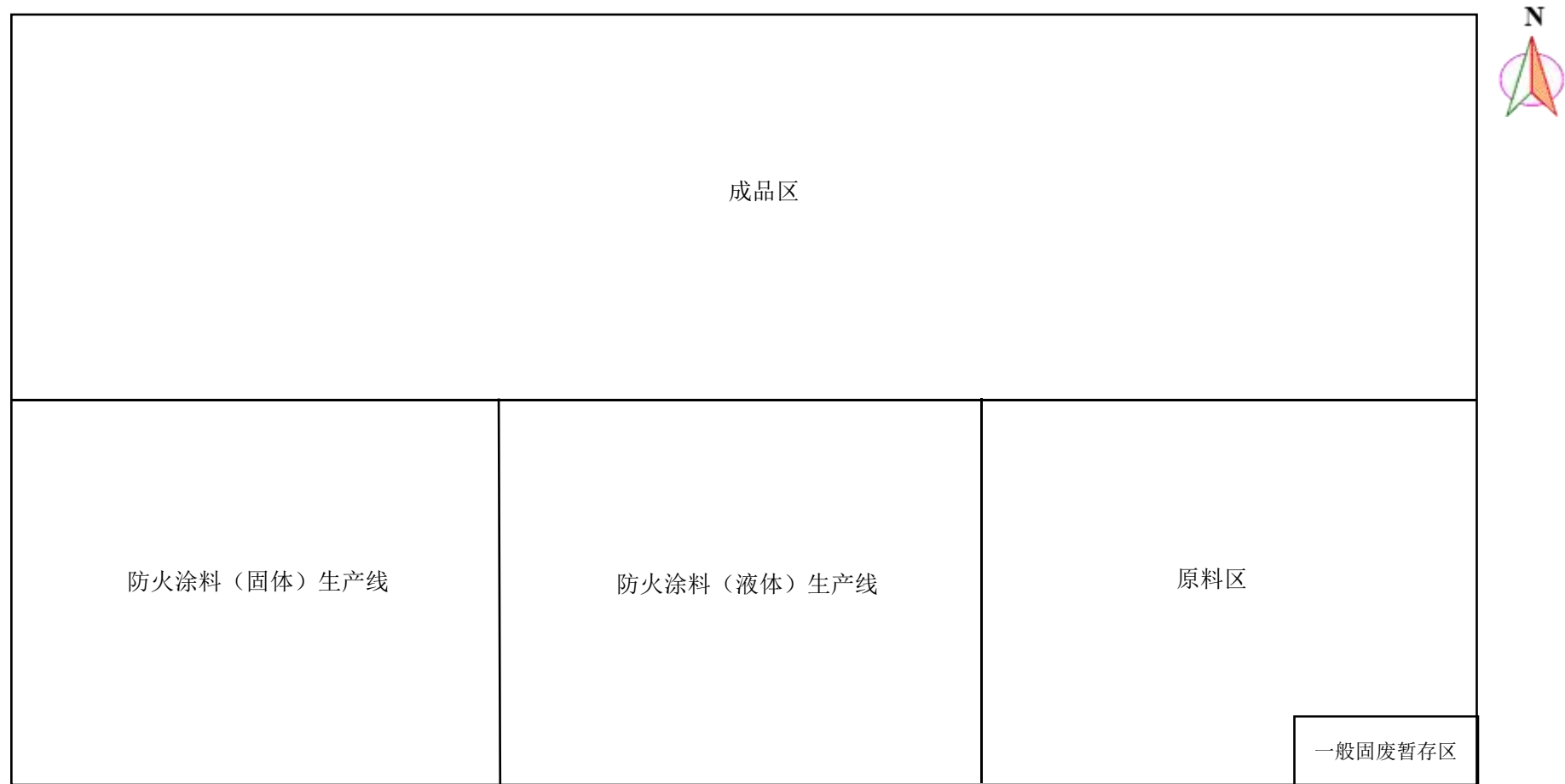
附图 4 项目生产车间布局图 （比例尺 1:500）
